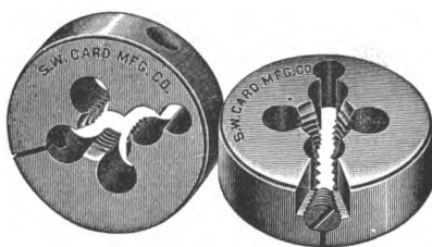
FIG. 47. DIES
